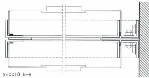
SECCIÓ B-B 1 / 2
