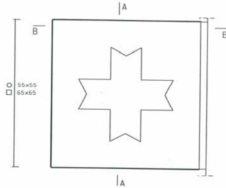
ALÇAT 1 / 10
