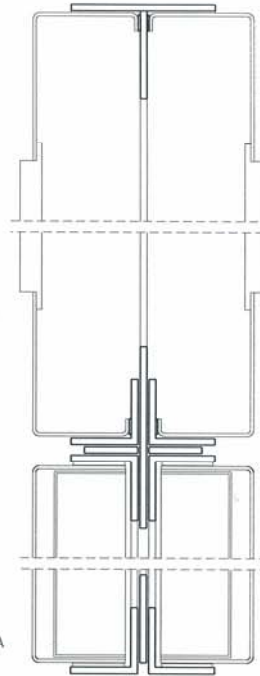
SECCIÓ A-A 1 / 2
