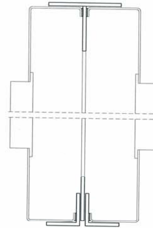
SECCIÓ A-A 1 / 2
