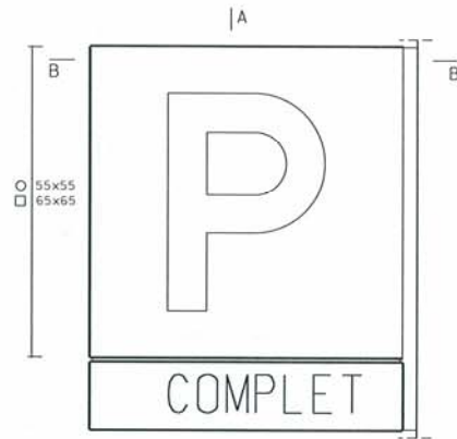
ALCAT 1 / 10
