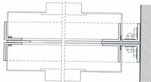
SECCIÓ B-B 1 / 2
